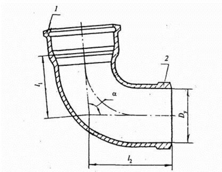
\alpha = 92^\circ 30' \pm 1^\circ 30' ; 1- раструб типа I; 2 - хвостовик
