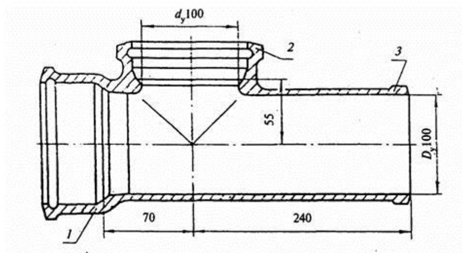
1 - раструб типа I; 2 - раструб типа IV; 3 - хвостовик
