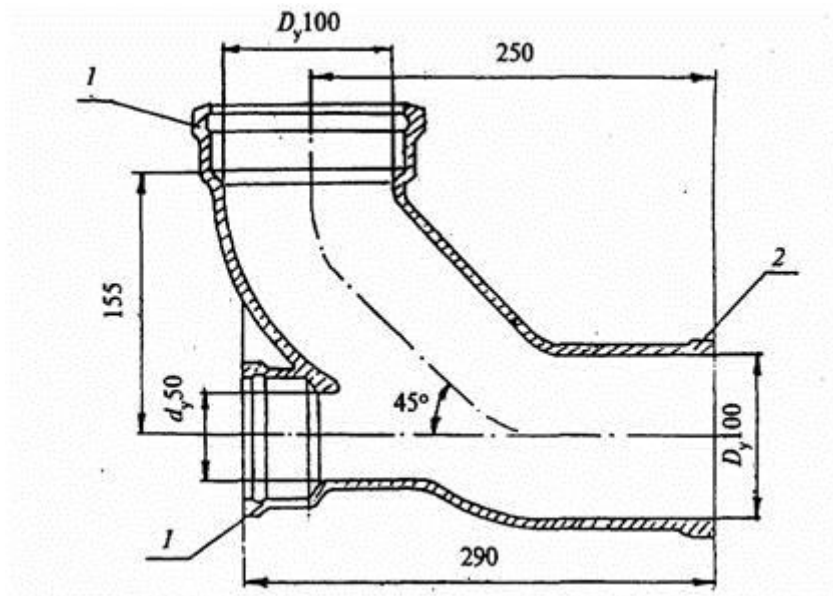
1 - раструб типа I; 2 - хвостовик
