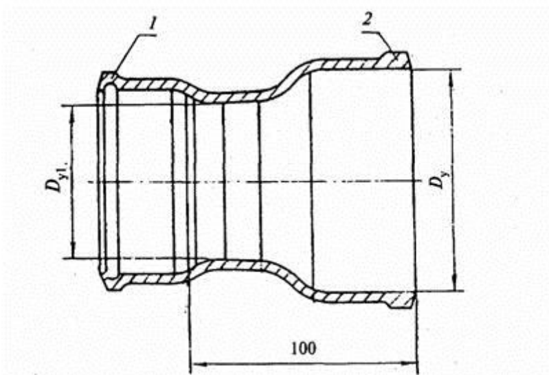
1- раструб типа I; 2 - хвостовик
