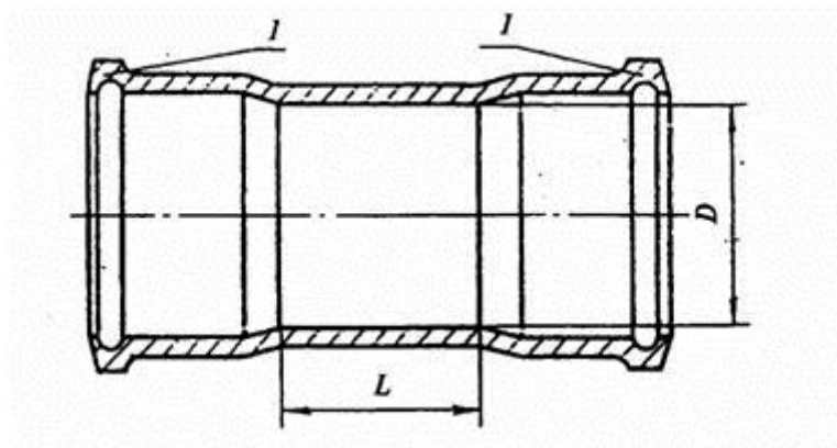
1 - раструб типа II
