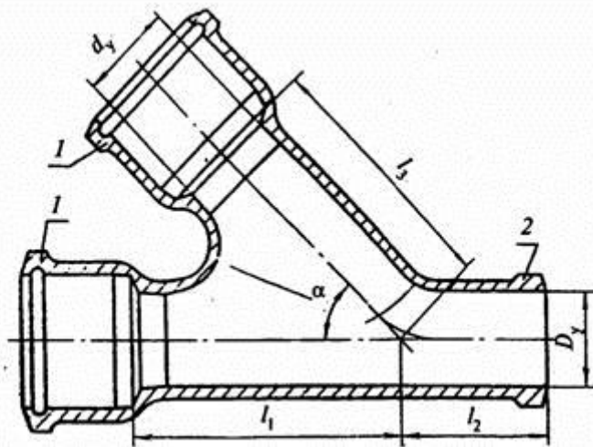
1 - раструб типа I; 2 - хвостовик
