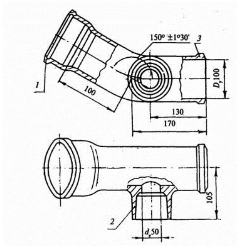
1 - раструб типа I; 2 - раструб типа III; 3 - хвостовик
