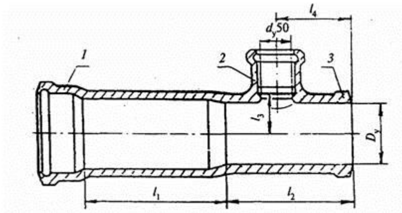
1 - раструб типа II; 2 - раструб типа I; 3- хвостовик
