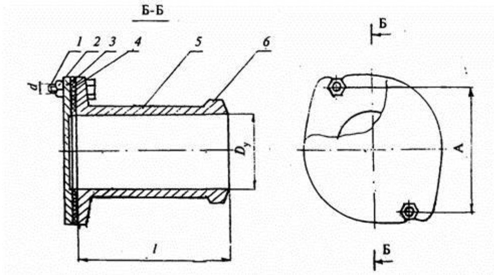
1- болт; 2 - гайка; 3 - крышка; 4 - прокладка; 5 - корпус; 6 - хвостовик
