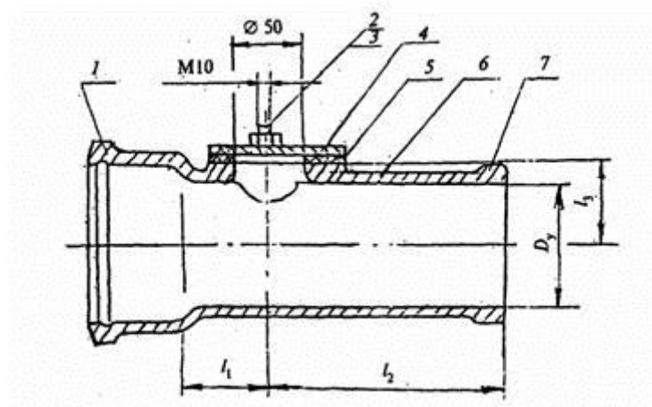
1 - раструб типа I; 2 - гайка; 3 - болт; 4 - крышка; 5 - прокладка;
