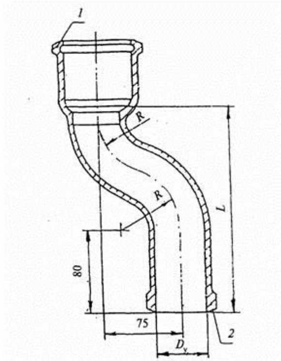
1 - раструб типа 1; 2 - хвостовик
