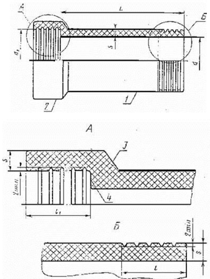
Керамическая канализационная труба
