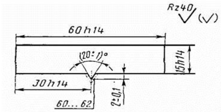
Шаблон для измерения глубины канавок
