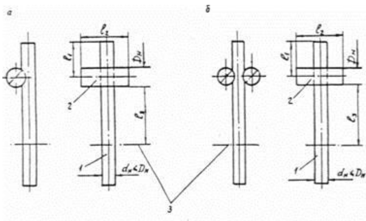
а с односрезное соединение; б с двухсрезное соединение; 1, 2 - стержни арматуры; 3 с граница закрепления в захвате разрывной машины
